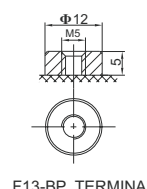
F13-BP TERMINAL
