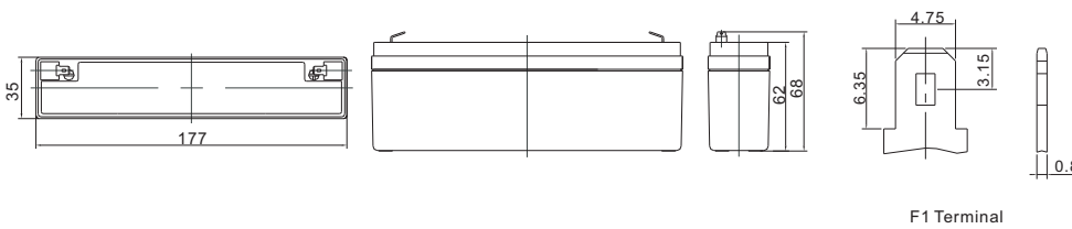
F1 Terminal
